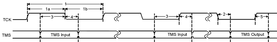
图 6-23cJTAG 时序
