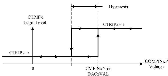
图 6-44CMPSS 比较器迟滞
