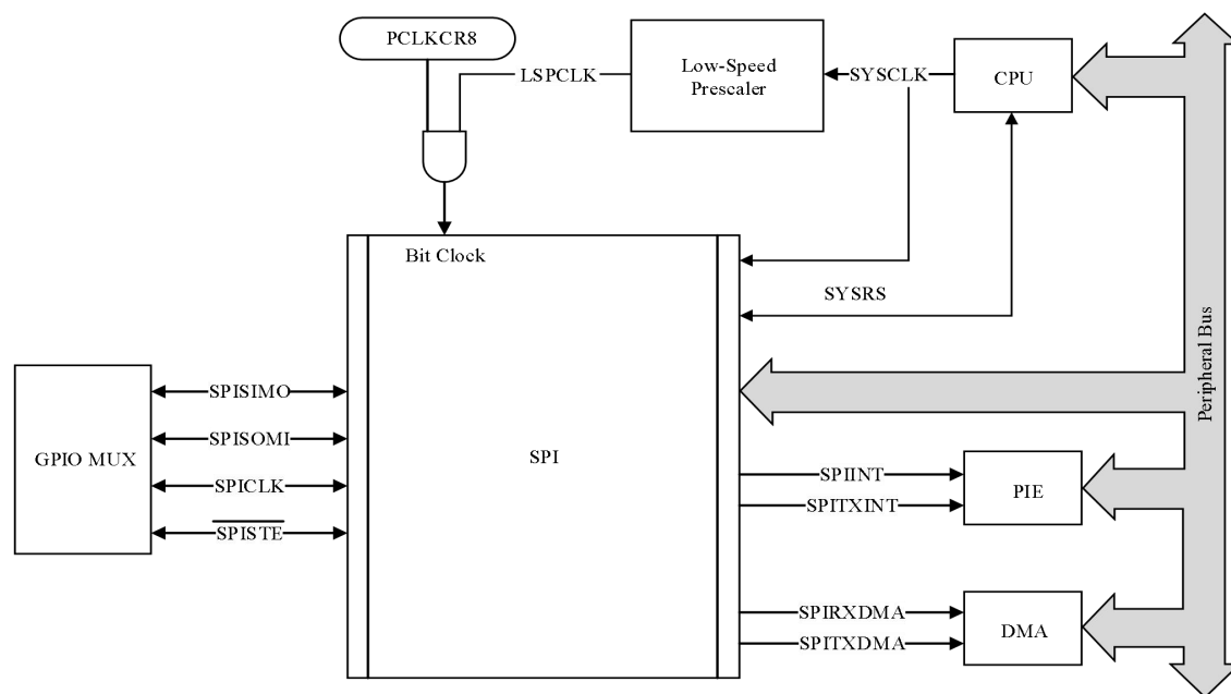
图 6-65 SPICPU 接口
