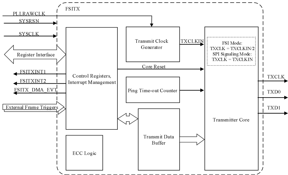
图 6-72FSITX 框图
