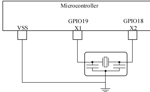
图 6-13 外部谐振器
