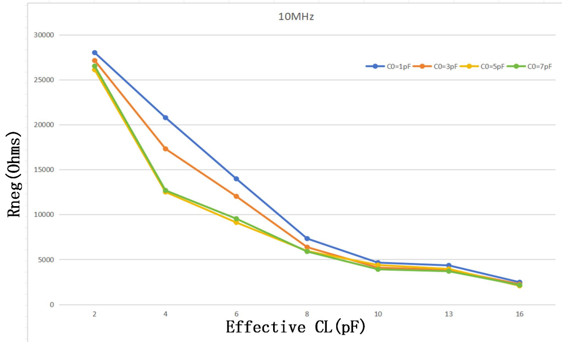
图 6-16. 10MHz 时的负电阻变化
