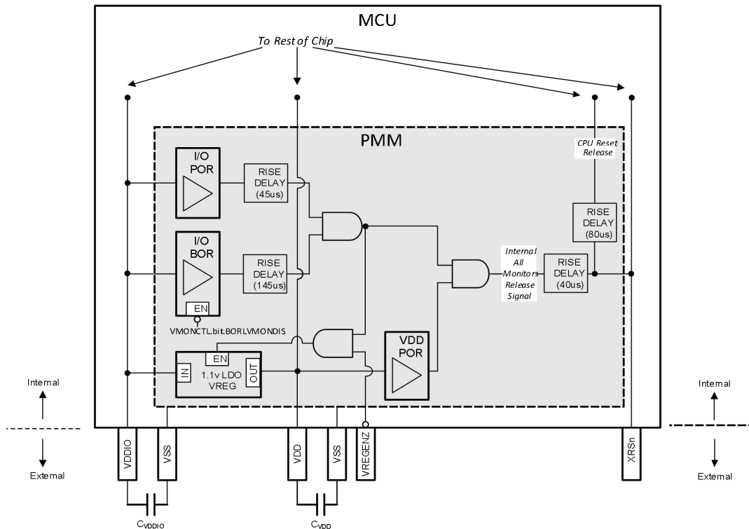
图 6-1PMM 框图
