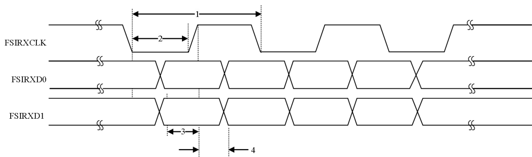
图 6-76FSIRX 时序
