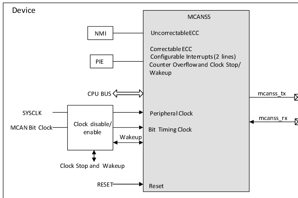
图 6-60MCAN 模块概述
