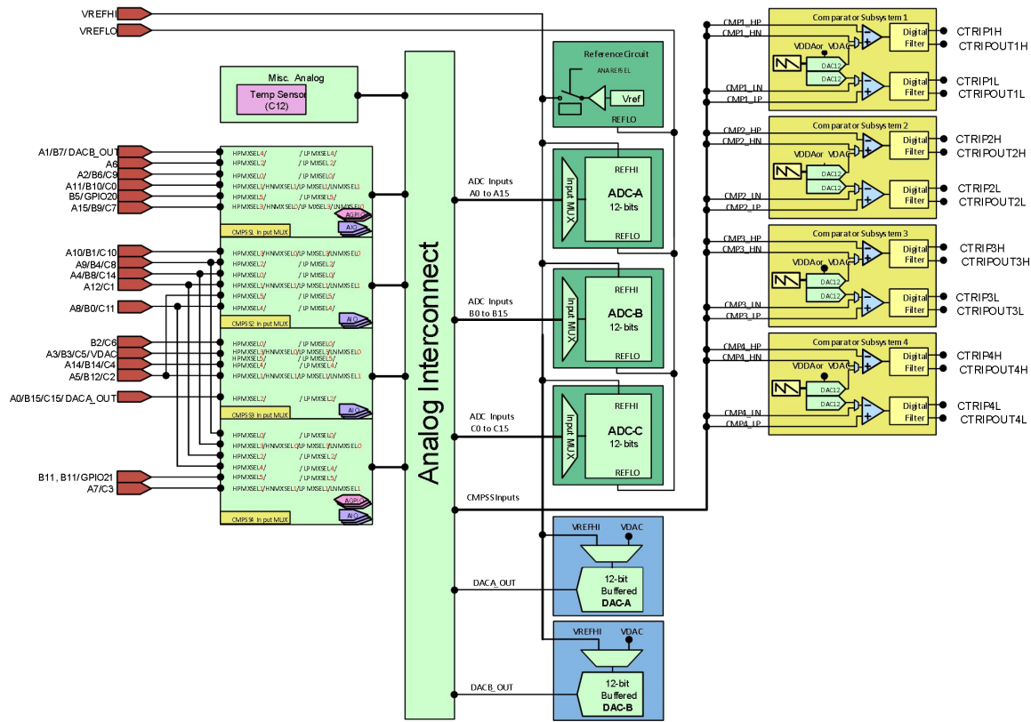
图 6-33 模拟子系统方框图 (80 引脚 LQFP)
