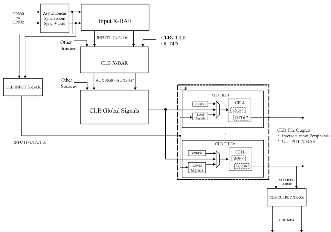
图 7-5GPIO 到 CLB 逻辑块的连接
