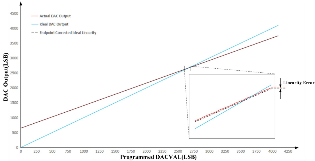
图 6-47CMPSS DAC 静态线性
