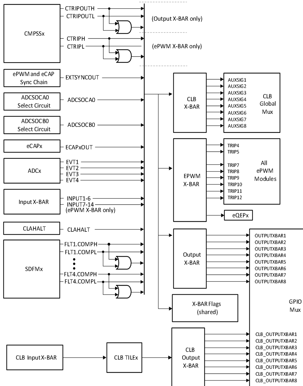
图 5-6 输出 X-BAR、CLBX-BAR、CLB 输出 X-BAR 和 ePWMX-BAR 源
