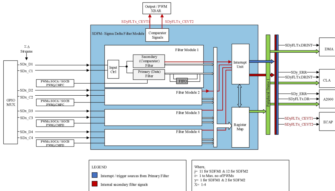
图 6-58Σ-Δ滤波器模块(SDFM)方框图
