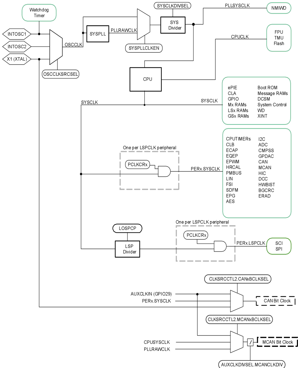
图 6-9 时钟系统
