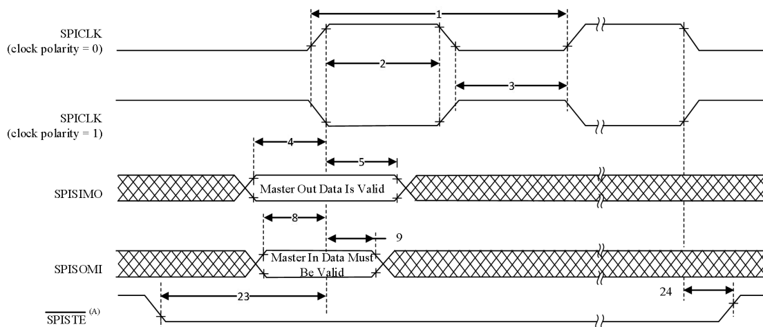
图 6-67SPI 主模式外部时序 (时钟相位=1)
