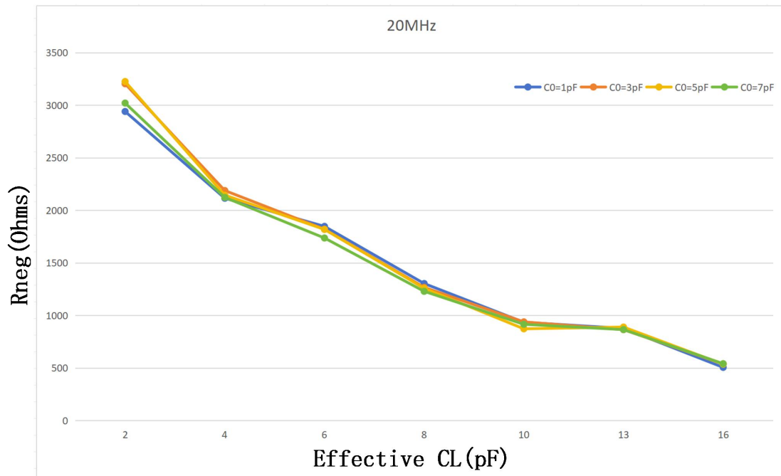
图 6-17. 20MHz 时的负电阻变化
