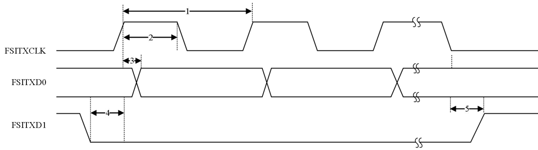
图 6-77FSITXSPI 信令模式时序
