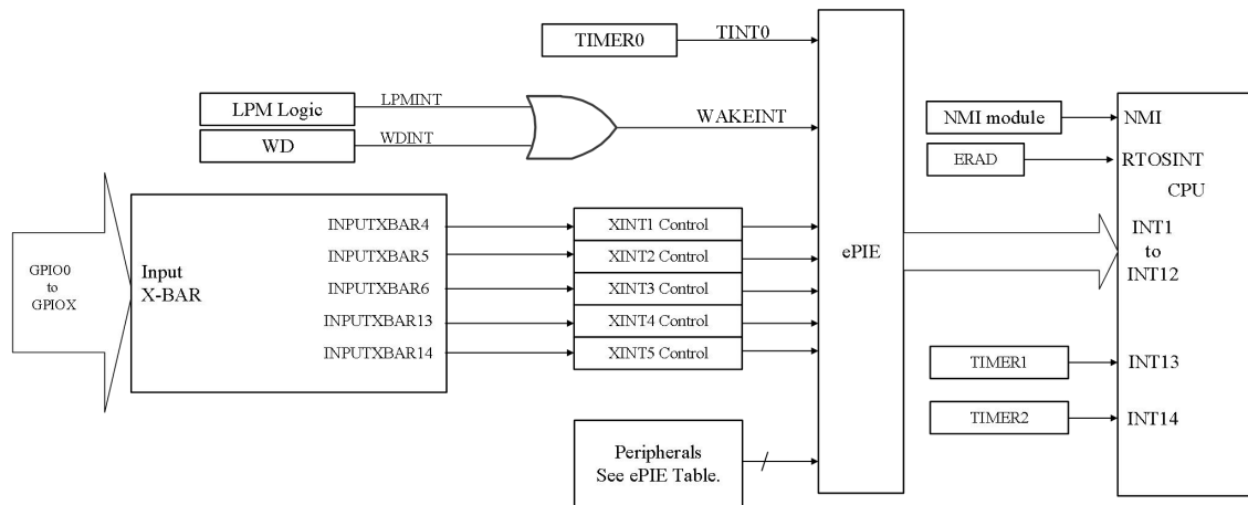
图 6-27 器件中断架构
