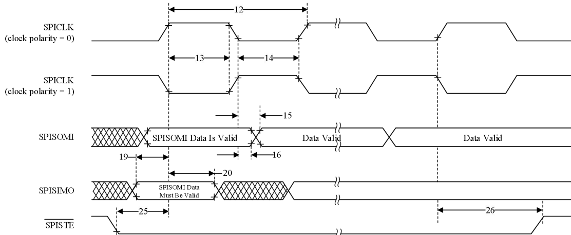
图 6-69 SPI 从模式外部时序 (时钟相位=1)
