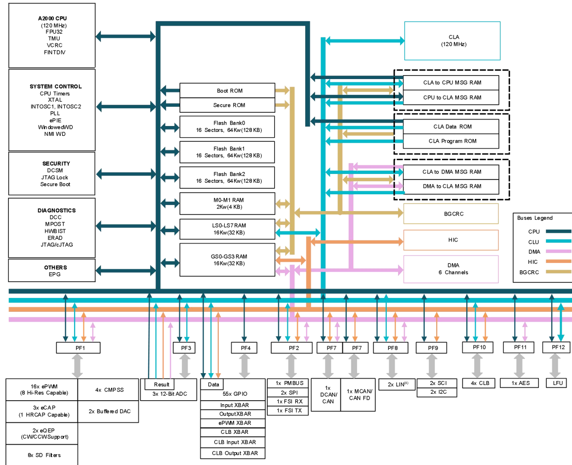
图 7-1 功能框图
