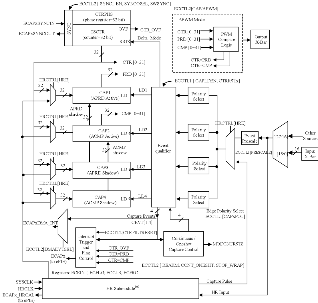
图 6-53eCAP 和 HRCAP 框图
