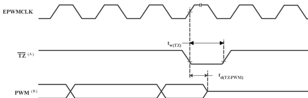
图 6-51 PWM 高阻态特征
