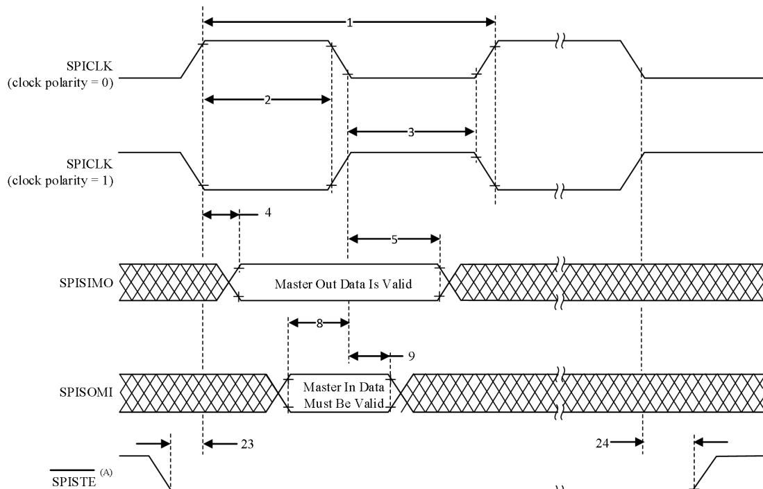
图 6-66SPI 主模式外部时序 (时钟相位=0)
