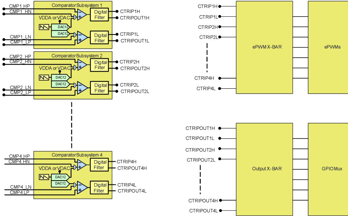
图 6-41CMPSS 连接
