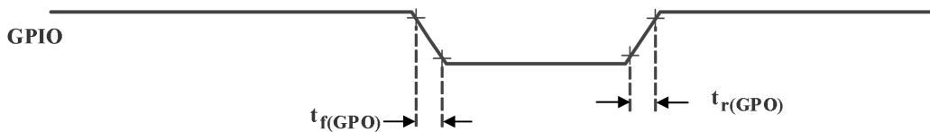
图 6-24 通用输出时序
