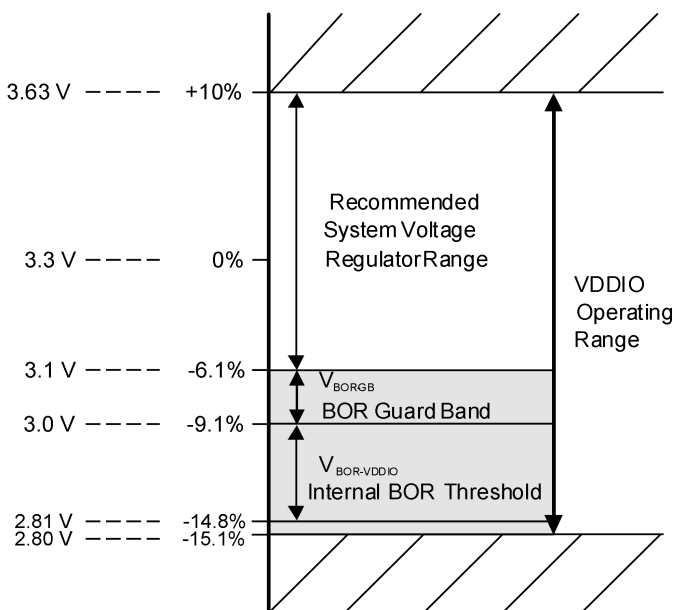
图 6-2 I/OBOR 工作区域
