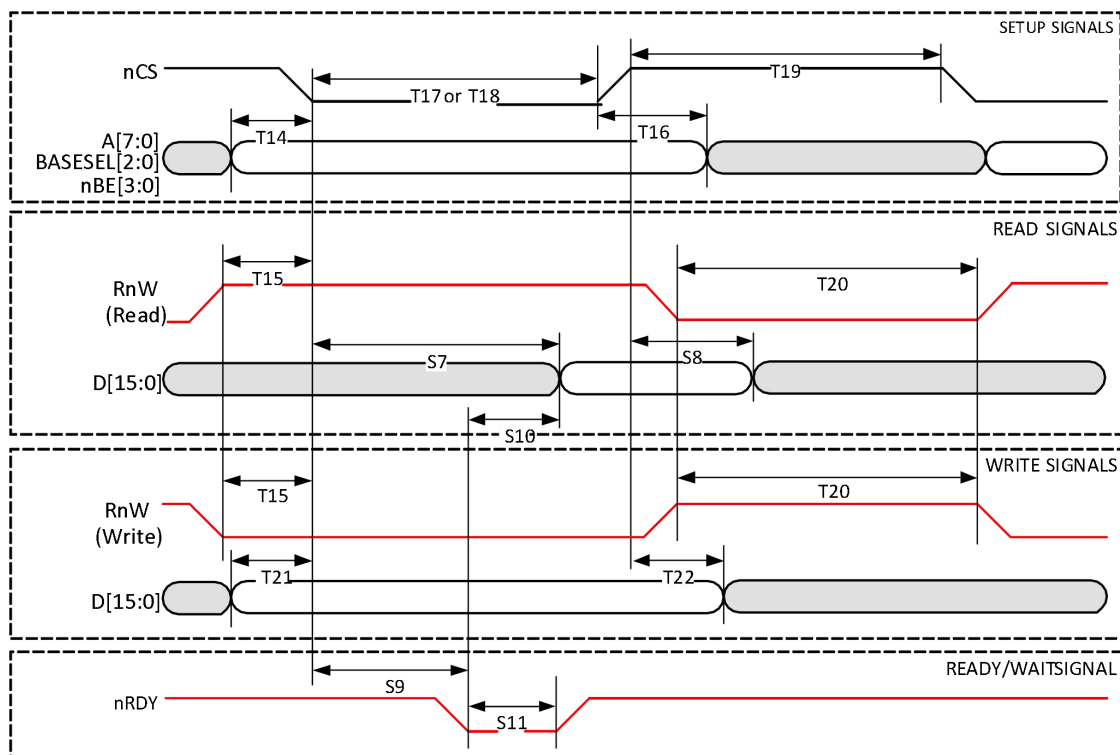
图 6-80 使用 RnW 引脚进行读取/写入操作
