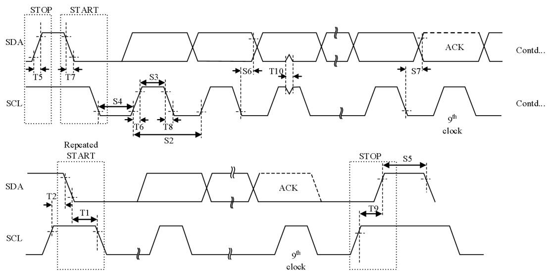
图 6-62I2C 时序图
