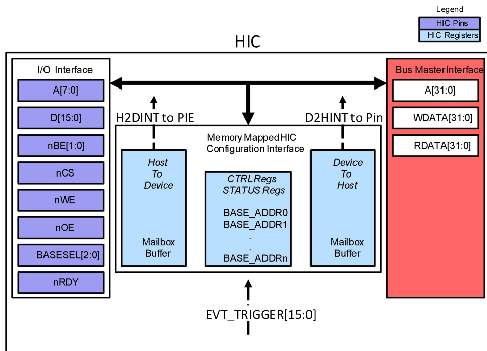
图 6-78 HIC 框图
