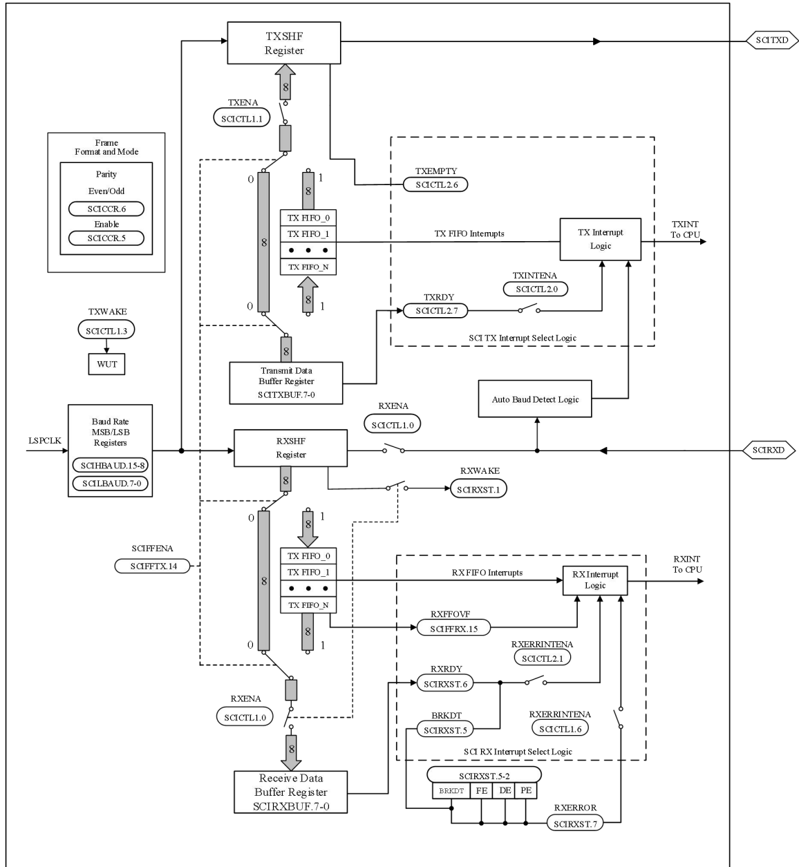
图 6-64SCI 框图
