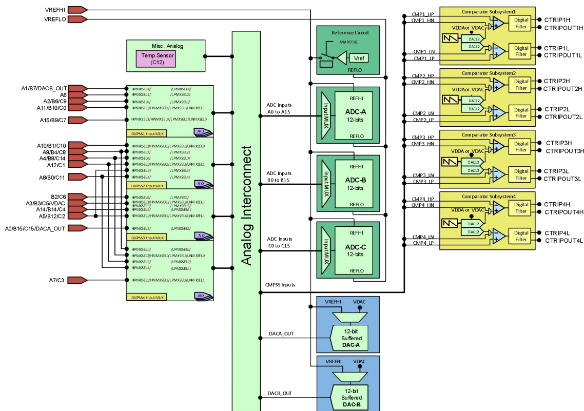
图 6-34 模拟子系统方框图 (64 引脚 LQFP)
