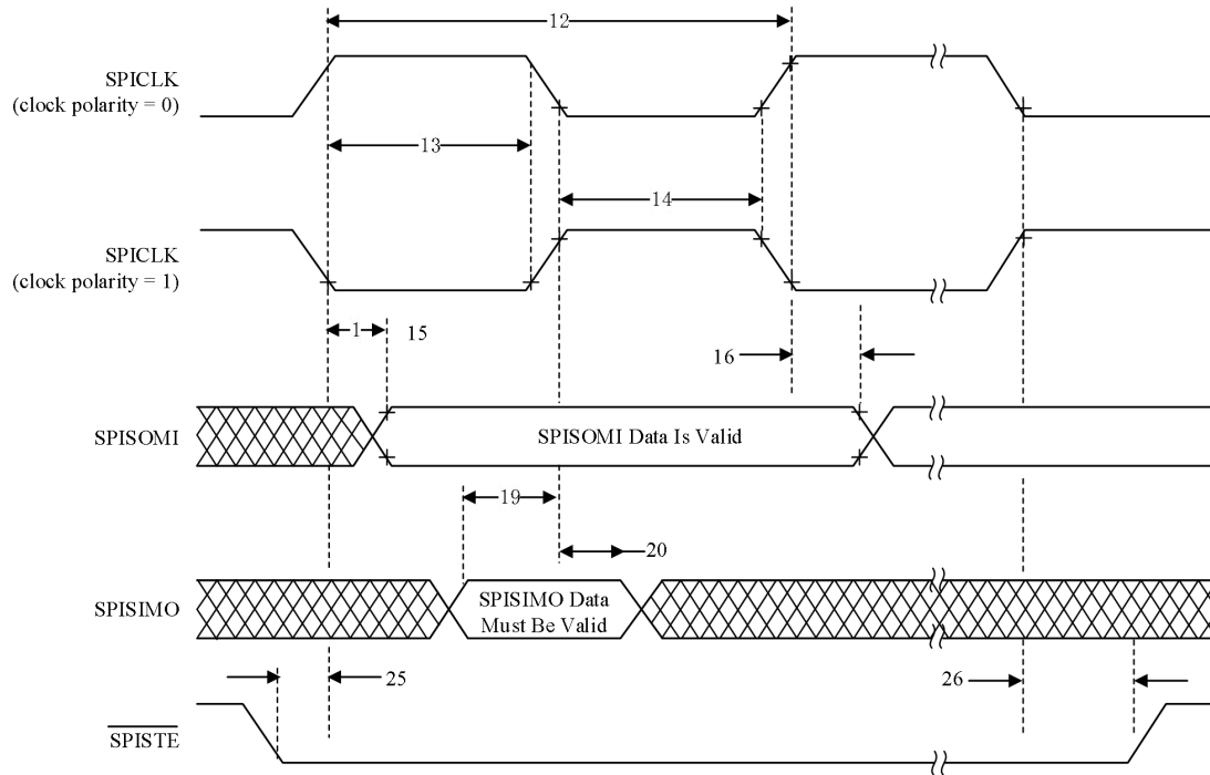
图 6-68 SPI 从模式外部时序 (时钟相位=0)
