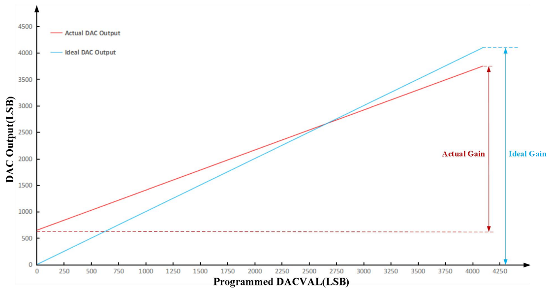
图 6-46CMPSS DAC 静态增益
