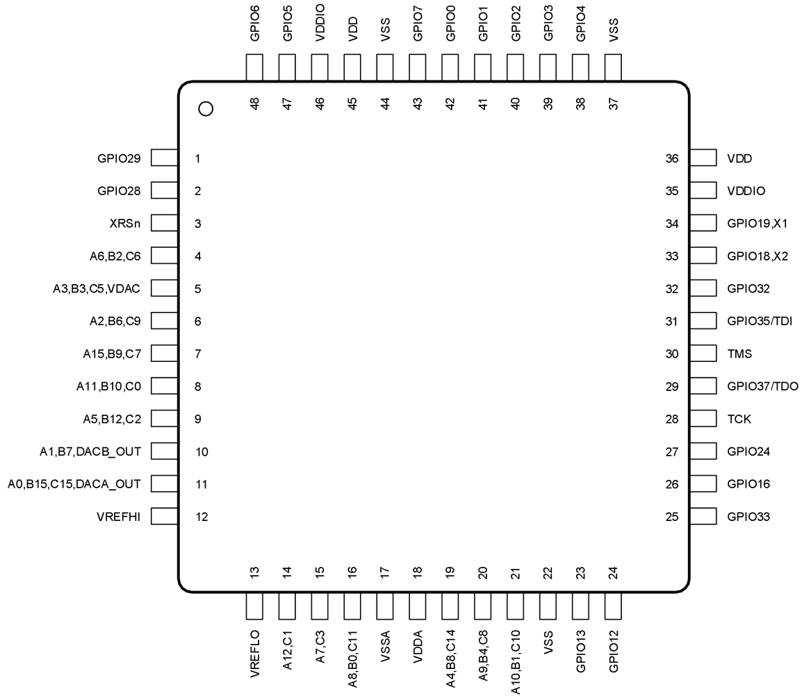
图 5-4 48 引脚 QP 薄型四方扁平封装 (AVP32F0025PQP48) (顶视图)
