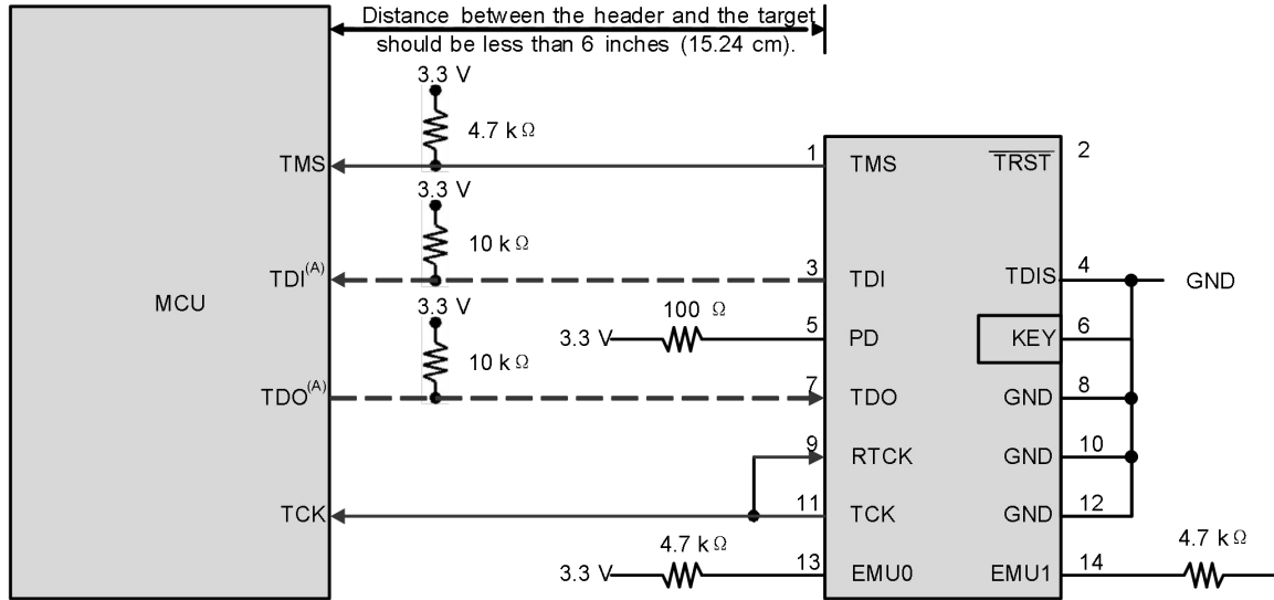
图 6-20 连接到 14 引脚 JTAG 接头
