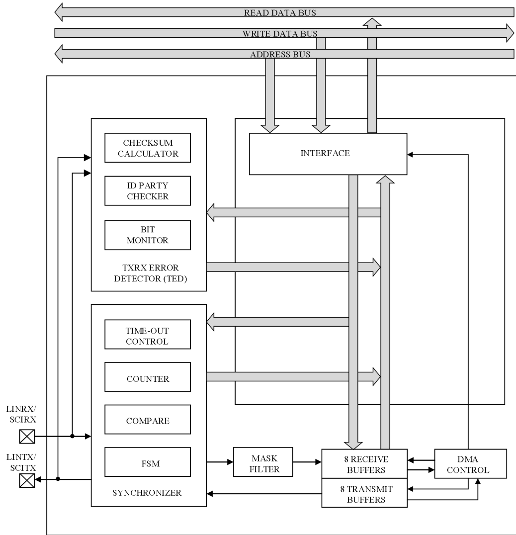
图 6-70LIN 框图
