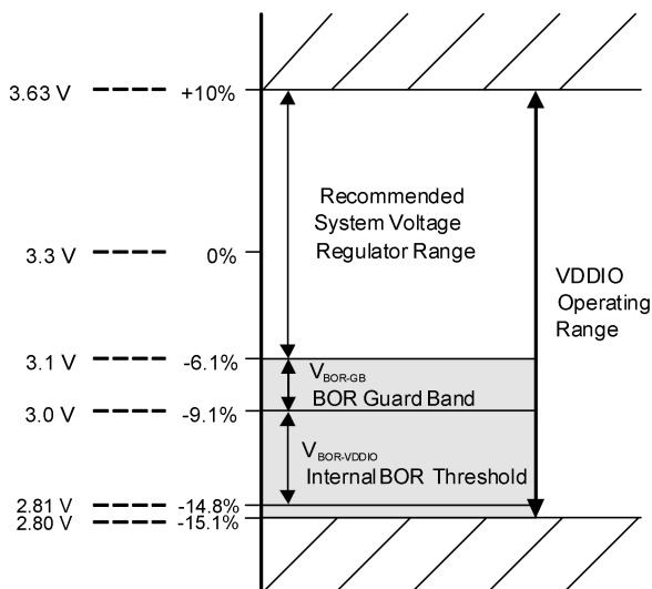
图 6-5 电源电压
