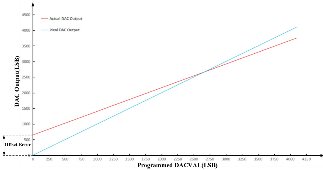
图 6-45CMPSS DAC 静态偏移量
