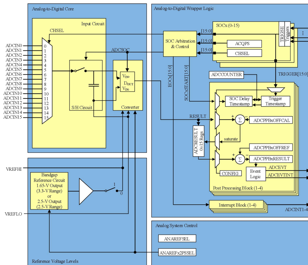
图 6-37ADC 模块方框图
