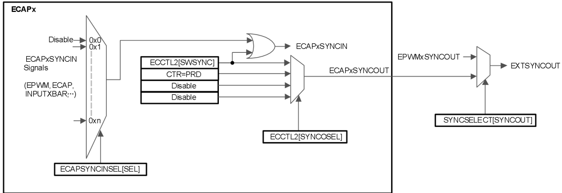
图 6-54eCAP 同步方案
