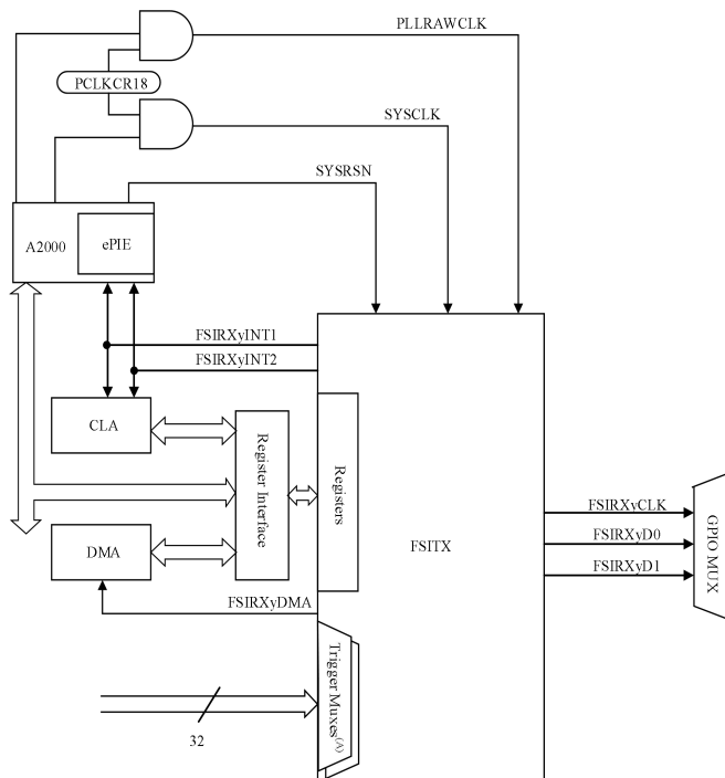
图 6-71FSITXCPU 接口
