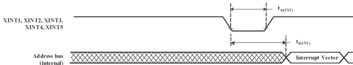
图 6-28 外部中断时序
