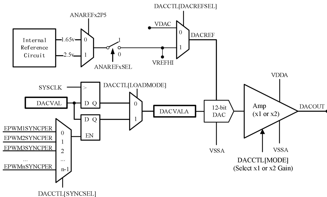
图 6-48DAC 模块框图
