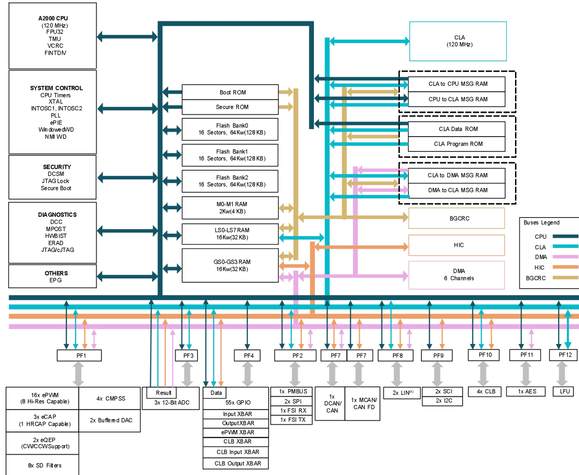
图 3-1 功能框图
