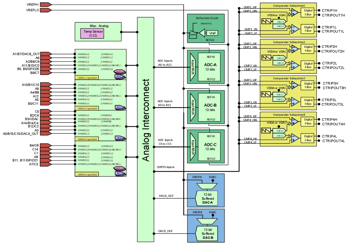
图 6-32 模拟子系统方框图 (100 引脚 LQFP)
