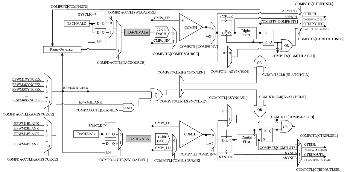
图 6-42CMPSS 模块框图
