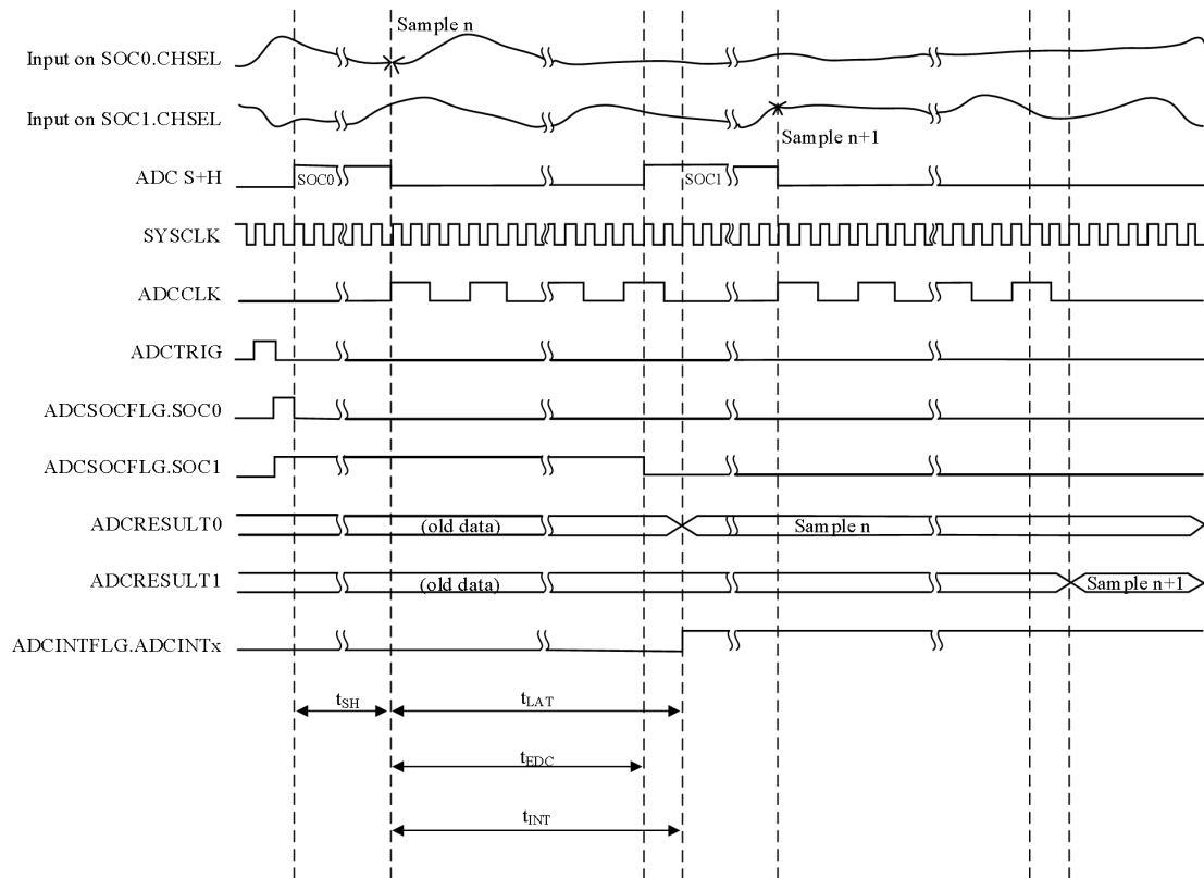
图 6-40ADC 时序
