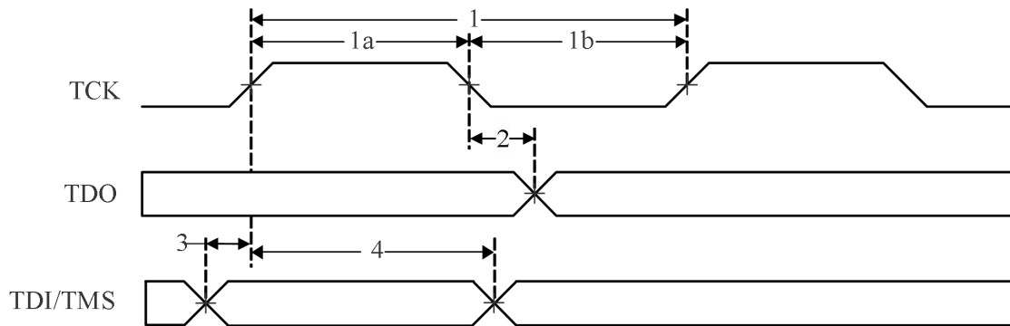
图 6-22JTAG 时序
