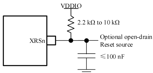
图 6-6 复位电路
