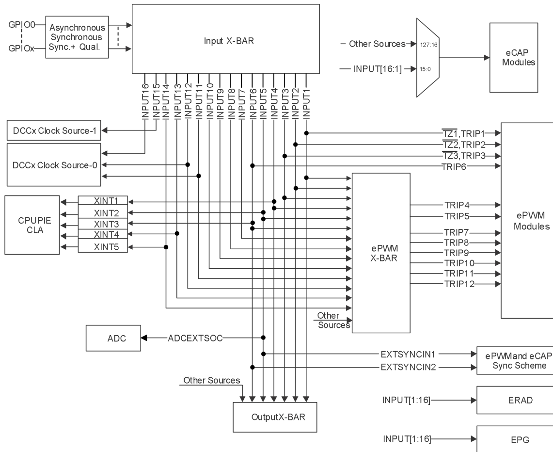
图 5-5 输入 X-BAR
