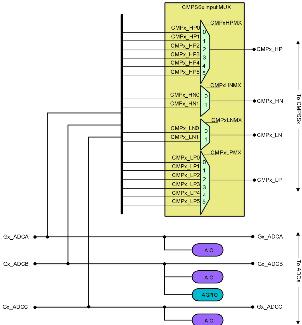
图 6-36 模拟组连接
