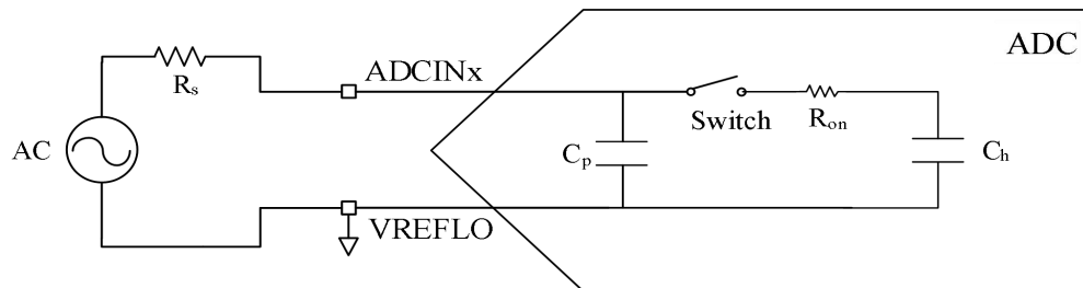
图 6-39 输入模型
