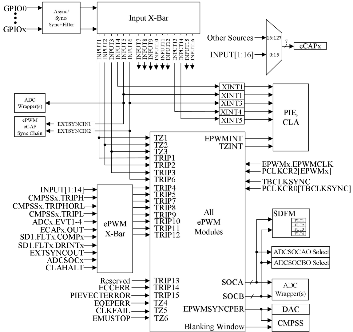
图 6-50ePWM 跳变输入连接
