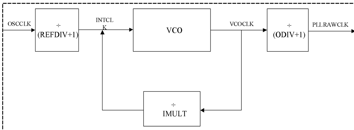
图 6-10 系统 PLL
