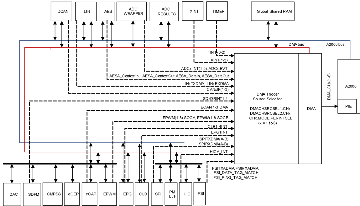
图 7-3DMA 框图
