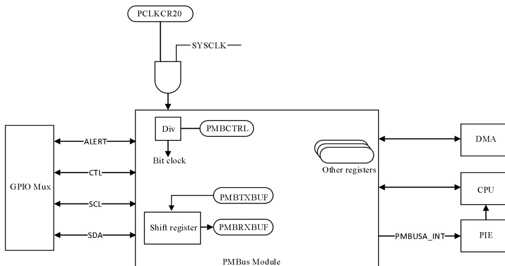
图 6-63PMBus 框图
