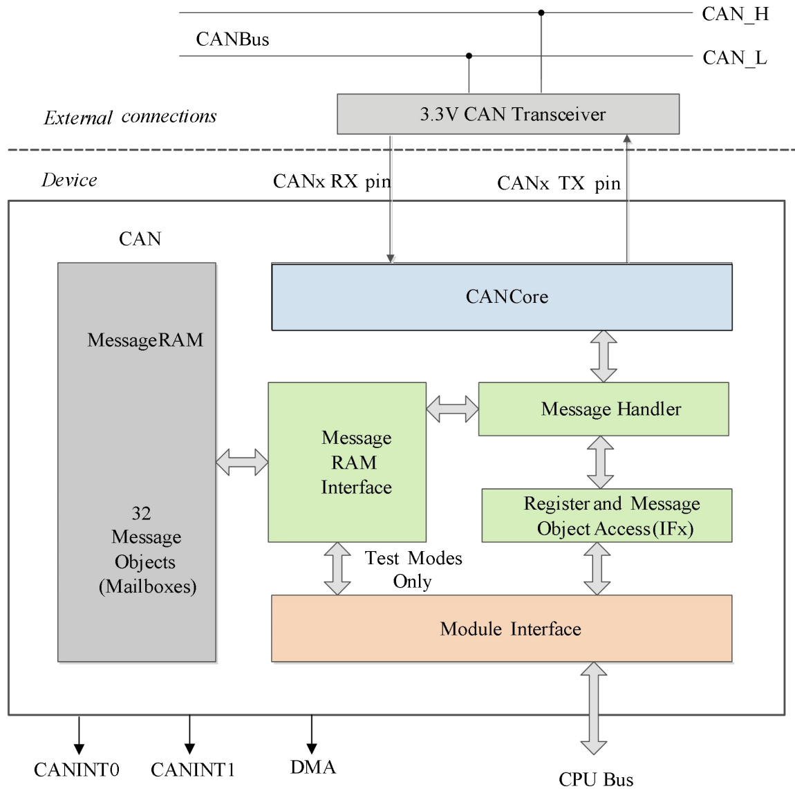
图 6-59CAN 框图
