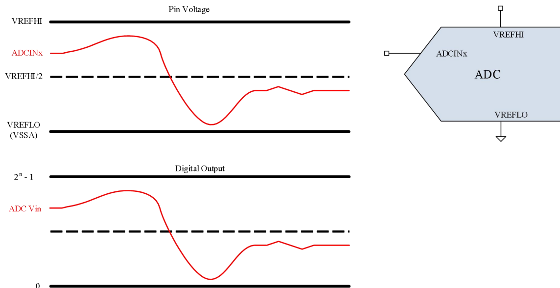
图 6-38 单端信号模式
